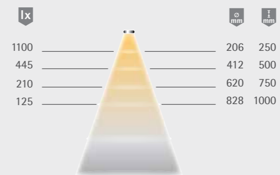
Lichtverteilungsdiagramm 45°
