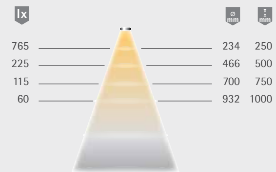
Lichtverteilungsdiagramm 50°
