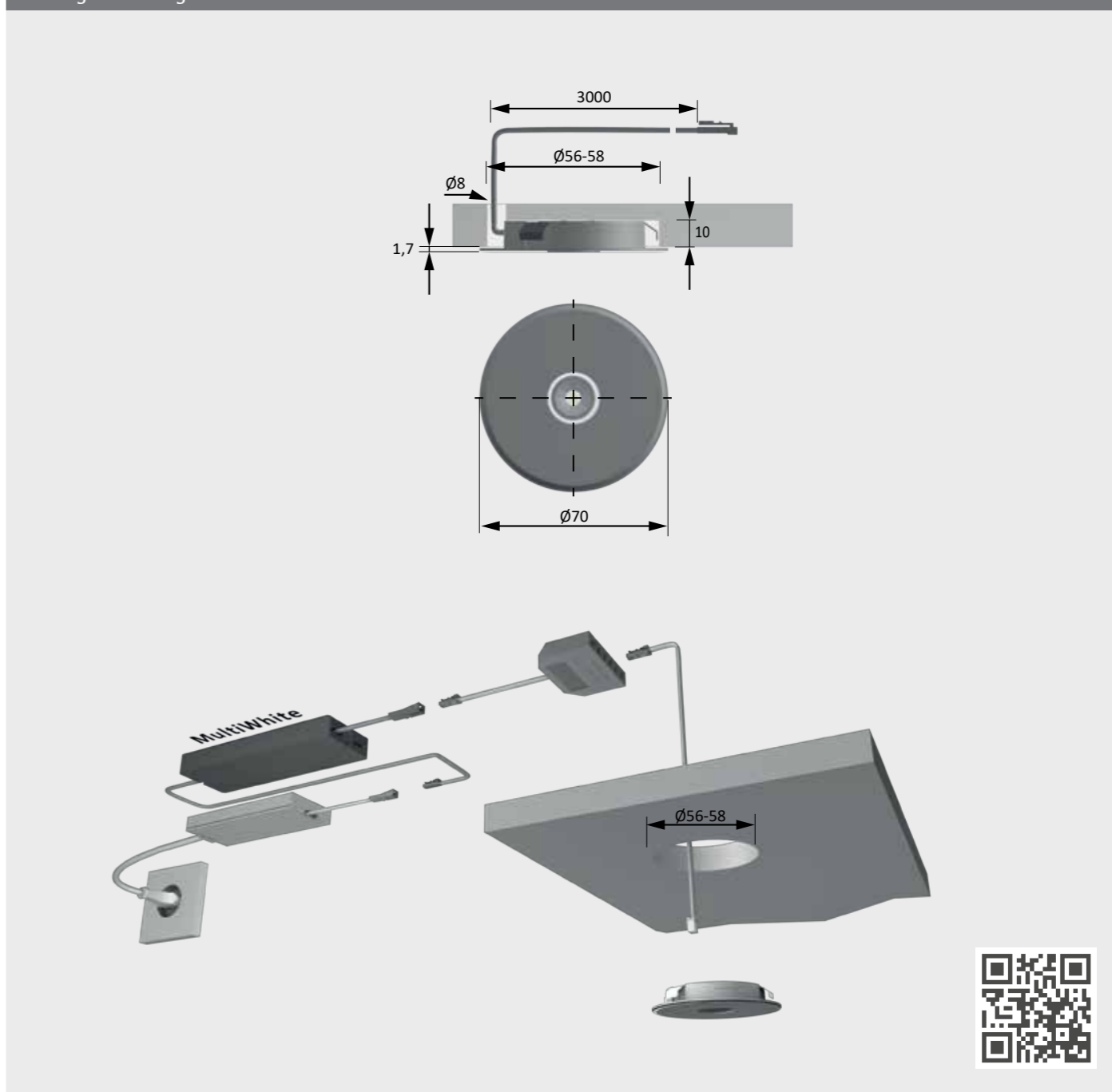
Montagezeichnung
